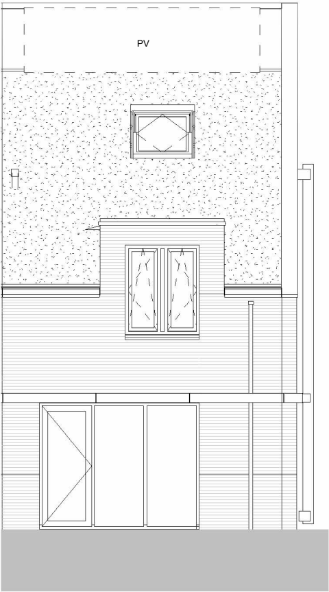
achtergevel
