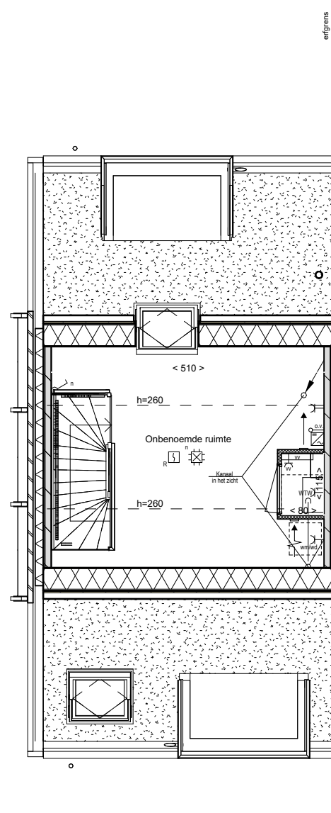
02 tweede verdieping
