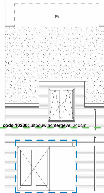
code 10800: dubbele openslaande deuren achtergevel
