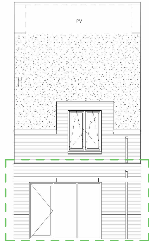
code 10100: uitbouw achtergevel 120cm
