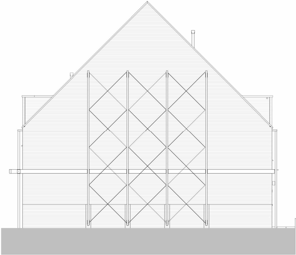
kopgevel
