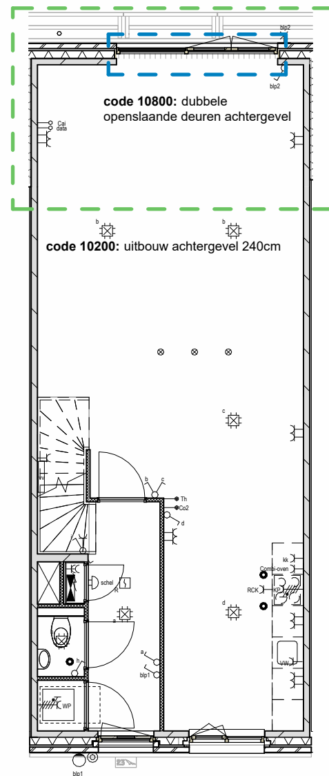
achtergevel
